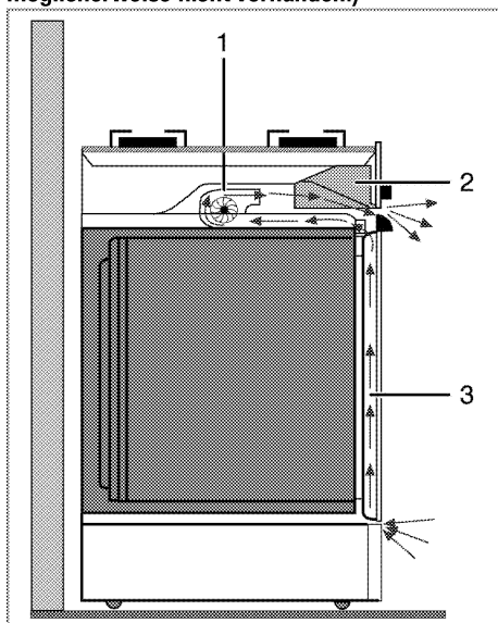
1 Lüfter
