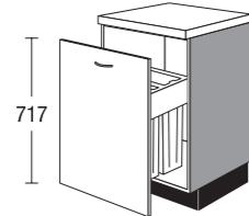
Unterschrank mit Wäschekörbe Höhe: 723 mm Breite: 500, 600 mm
